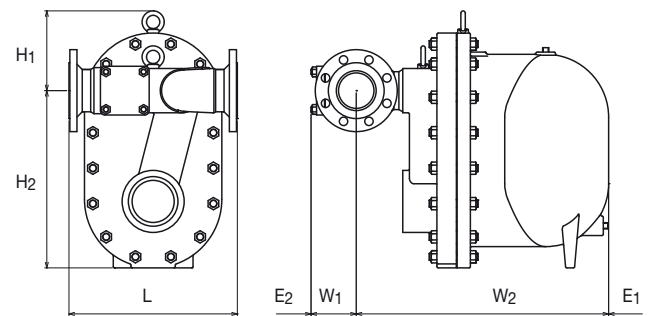
Dimensions GH70
